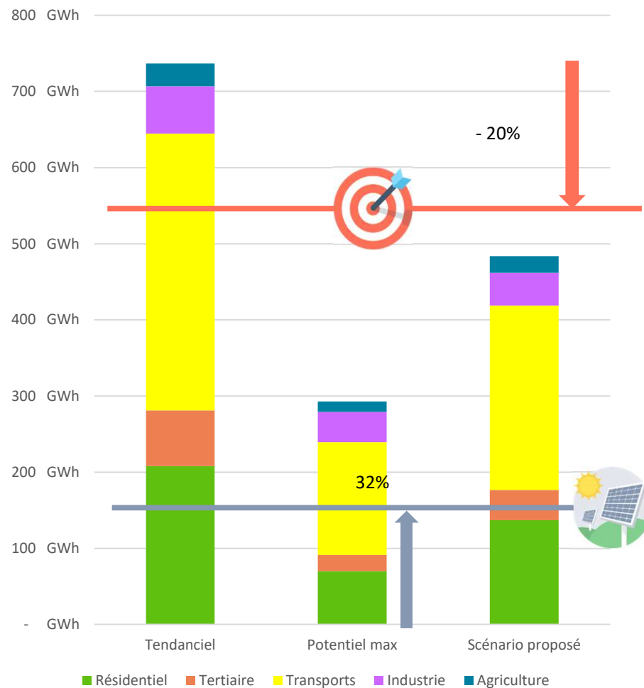
Consommations d'énergie en 2030 en fonction des scénarios
