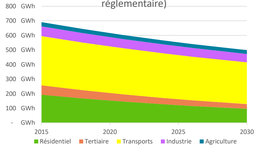
Consommation d'énergie finale (scénario réglementaire)
