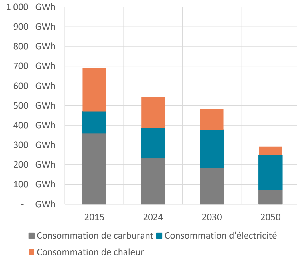
Evolution des consommations par vecteur énergétique
