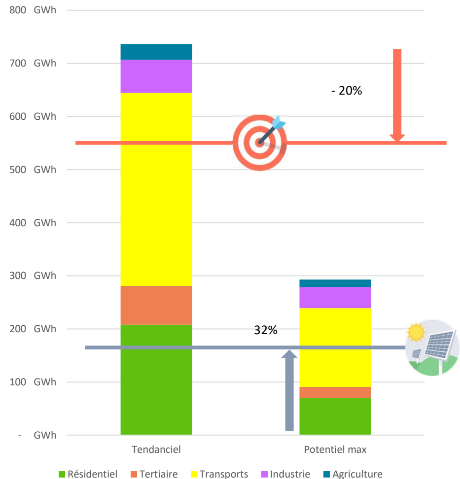
Consommations d'énergie en 2030 en fonction des scénarios
